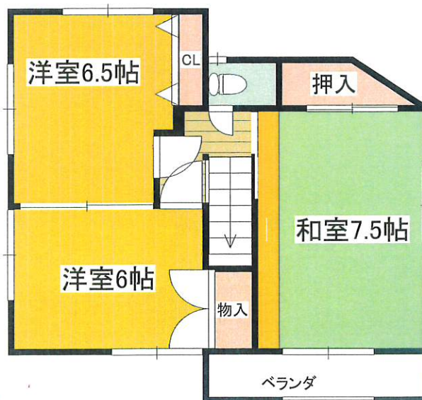
2階平面図
