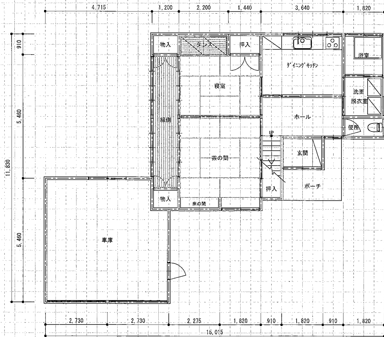
1階平面図 1/100
