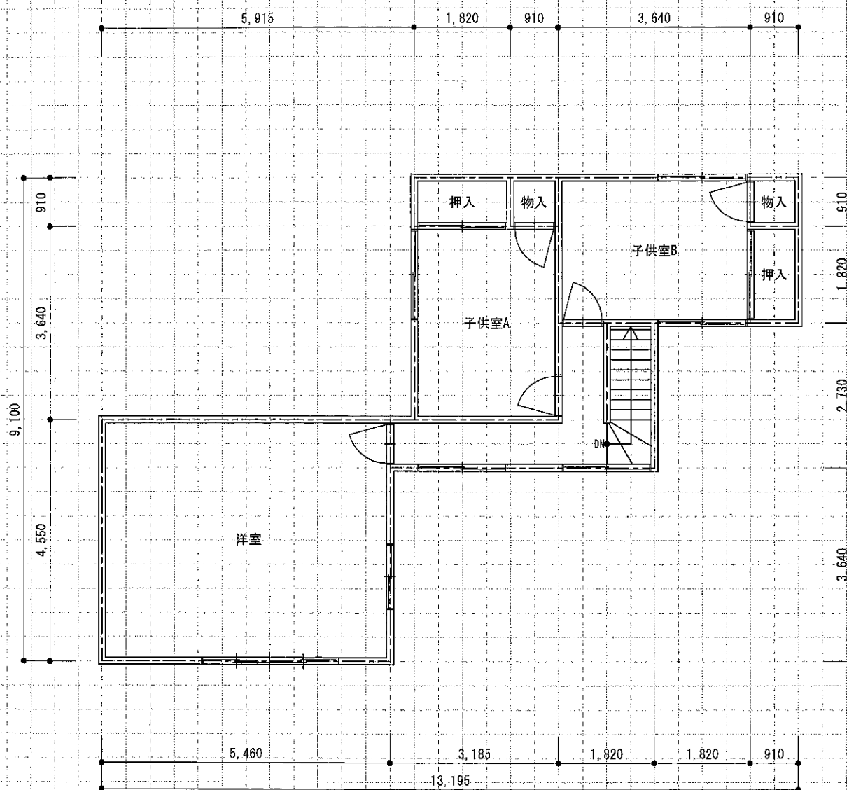
2階平面図 1/100
