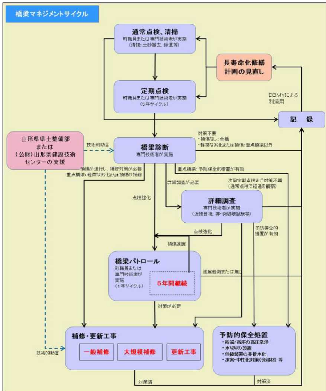
図-7 橋梁マネジメントフロー図
