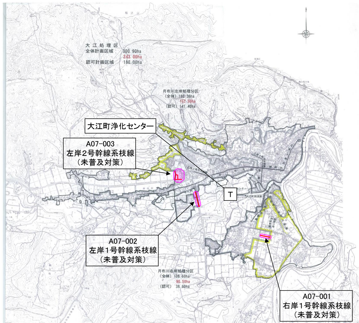
大江町処理区計画図
